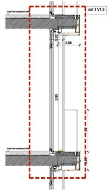
SECCIÓN V1.3
