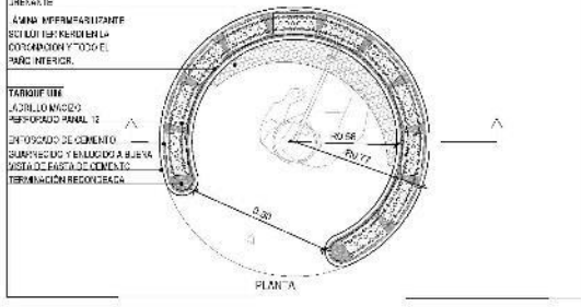
DETALLE DUCHA EXTERIOR
