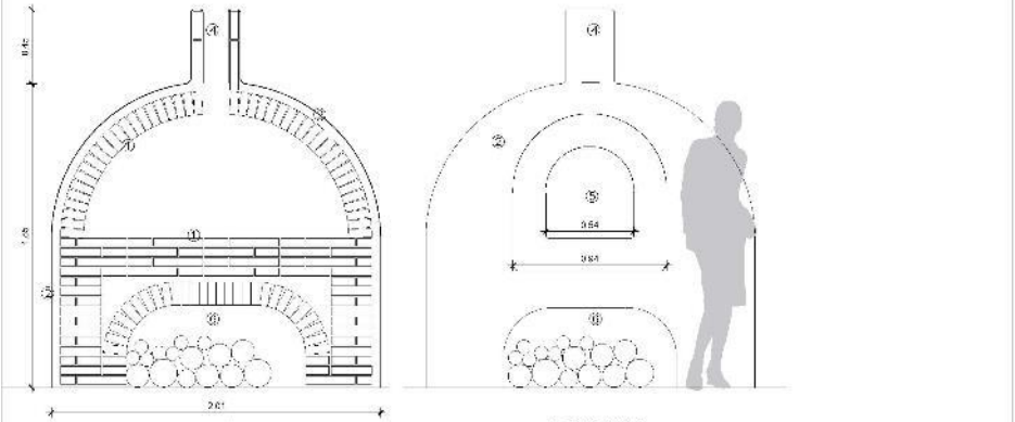
DETALLE HORNO DE LEÑA IBICENCO
