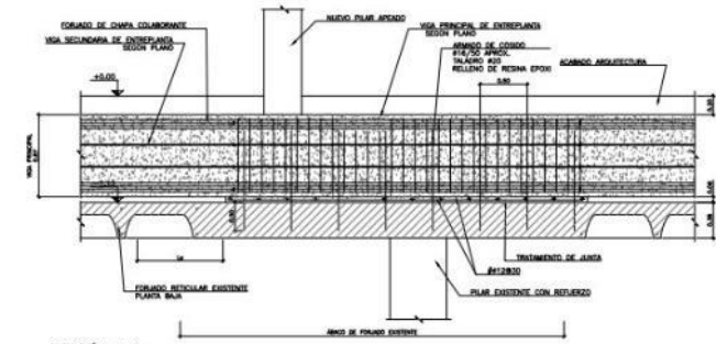
SECCIÓN A-A. DETALLE DE ARMADO DE NUDOS DE VIGAS PRINCIPALES SOBRE ÁBACO CON PILAR APEADO 1/20
